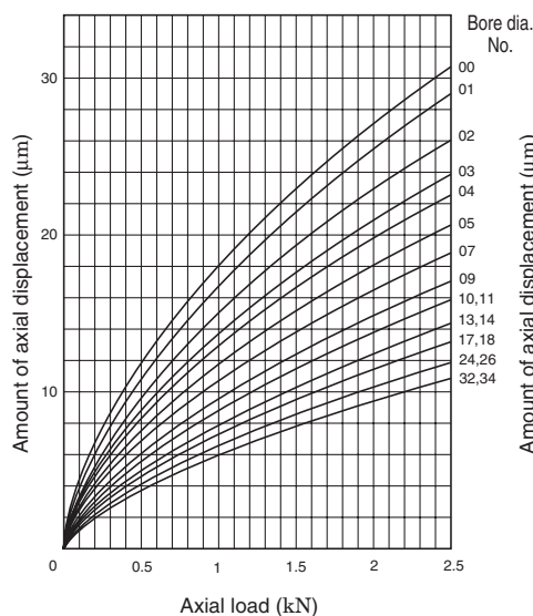
(4) 7000 (contact angle 30°)
